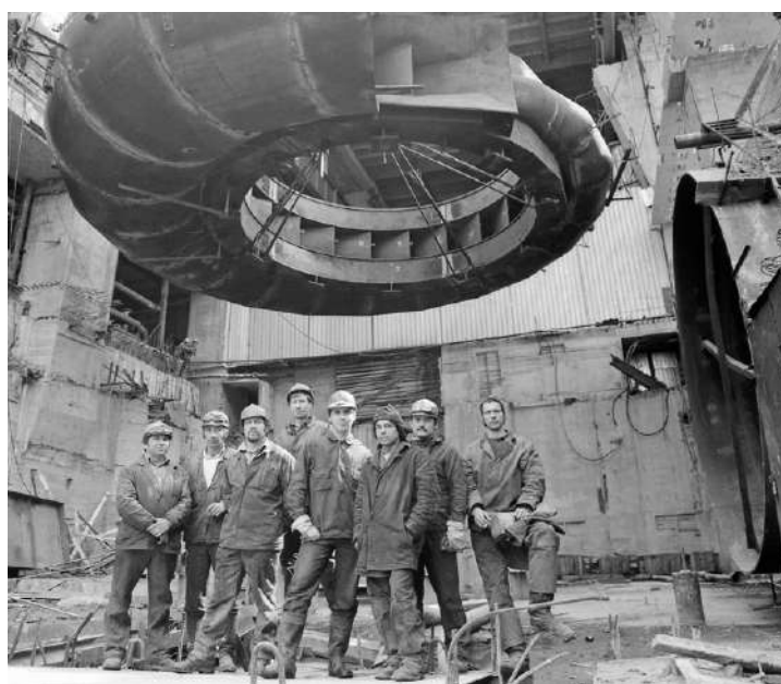
Бригада под спиральной камерой
